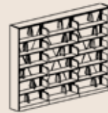
PLATO SO P3D1 / P3D2 L: 2769 mm D: 320 / 600 mm H: 2070 mm
